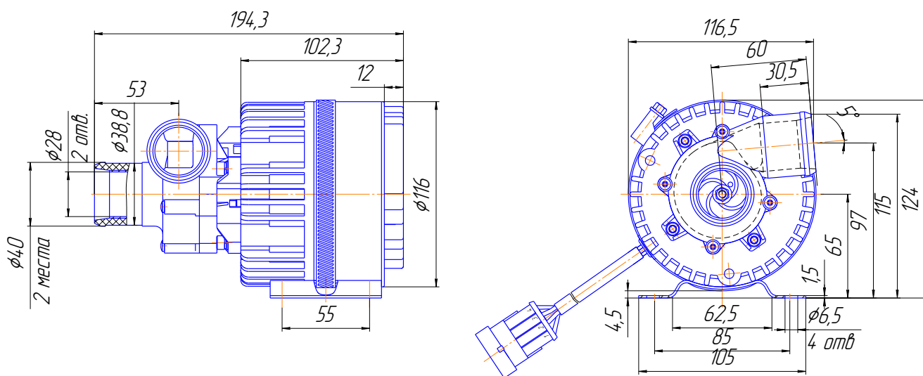
Рис.5 – Габаритные и установочные размеры помпы.
